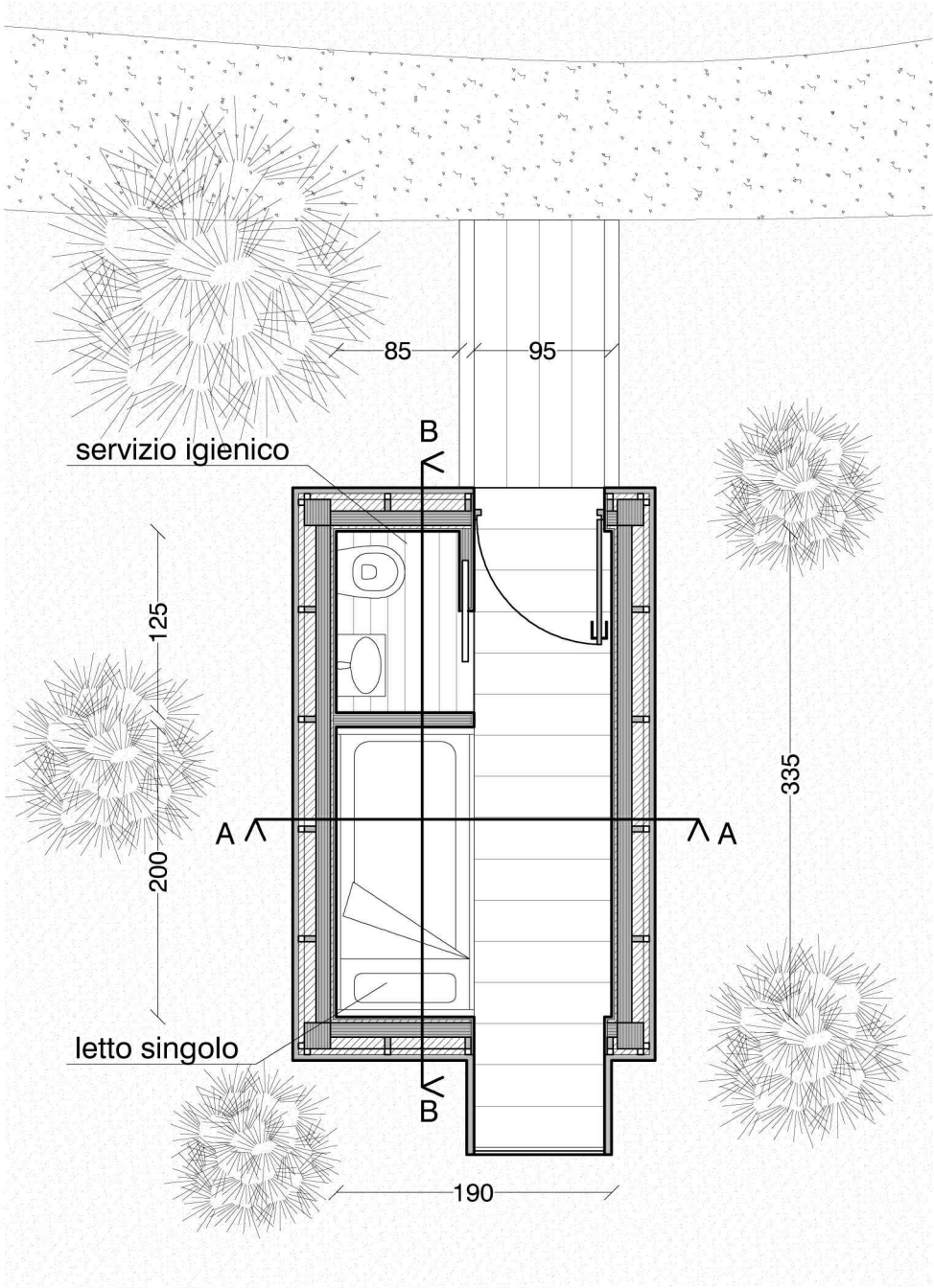
ALLOGGIO SINGOLO - PIANTA LIVELLO 0 Scala 1:50
