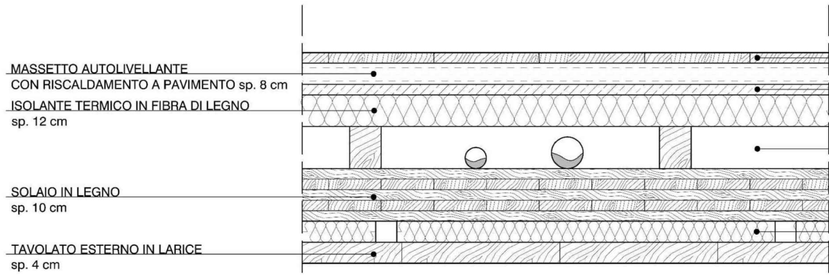
DETTAGLIO SOLAIO
