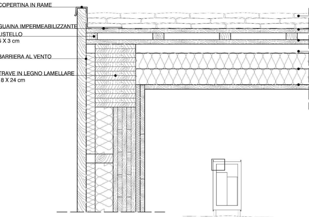
ALLOGGIO SINGOLO - DETTAGLIO NODO PARETE/COPERTURA Scala 1:10
