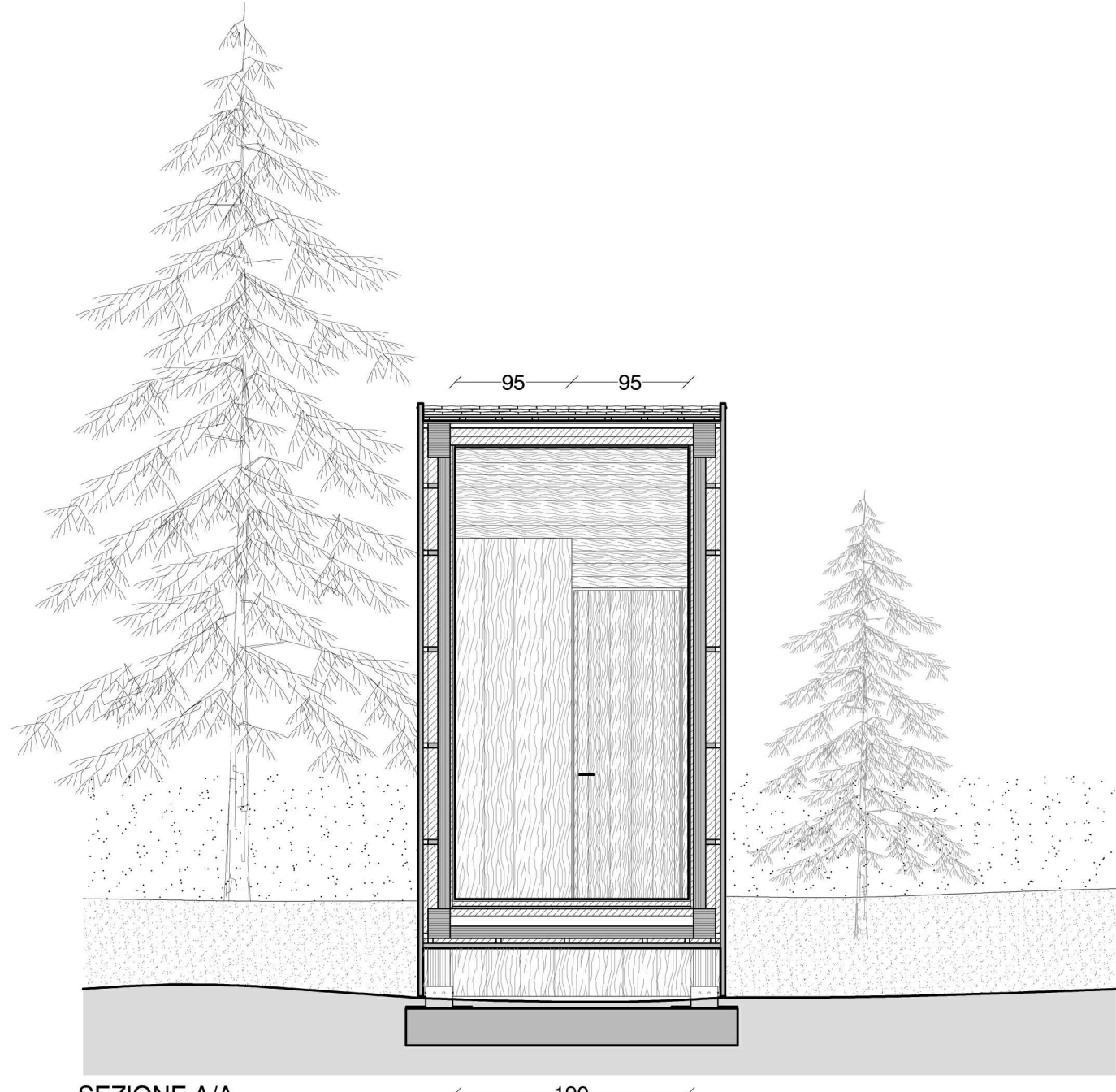
SEZIONE A/A
