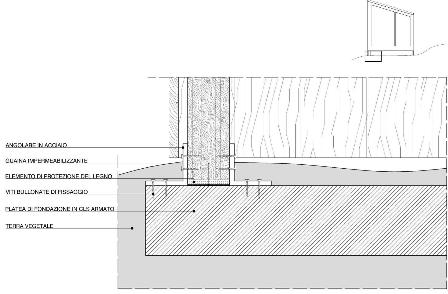
DETTAGLIO ATTACCO A TERRA
