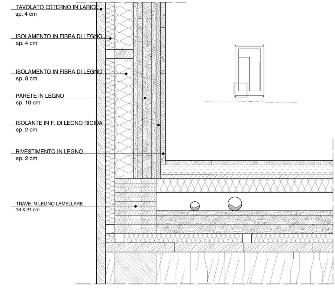
DETTAGLIO NODO PARETE/SOLAIO
