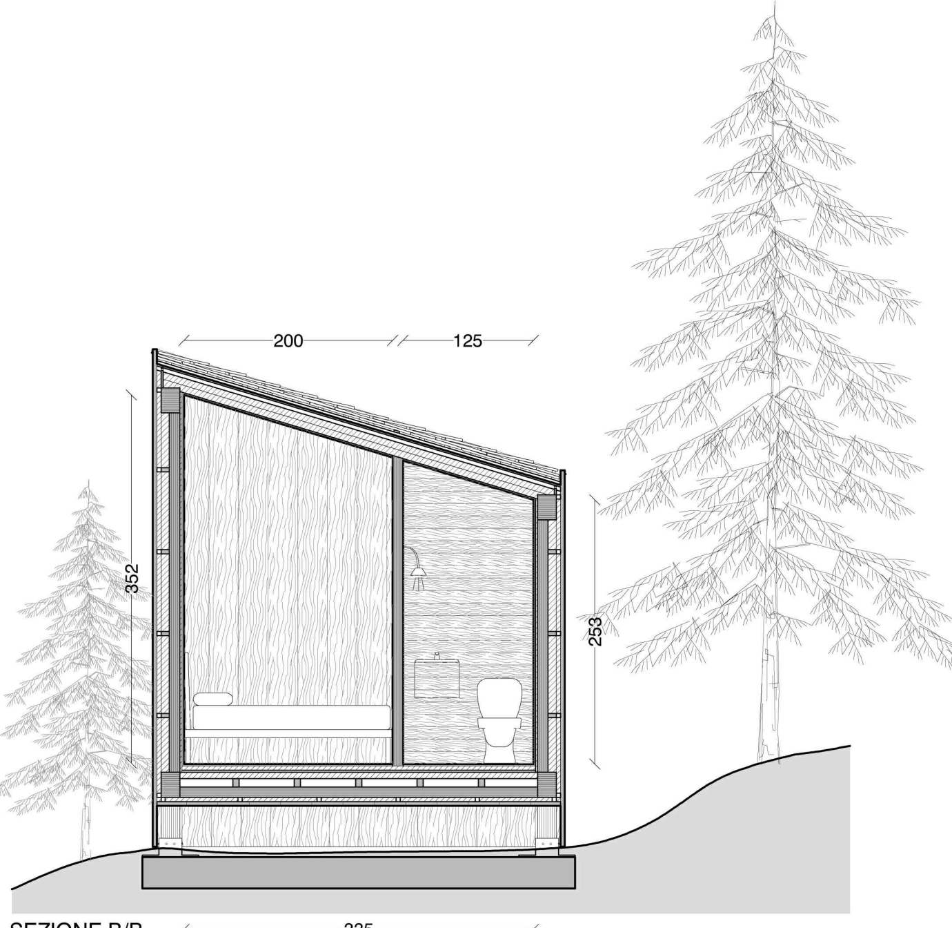
SEZIONE B/B
